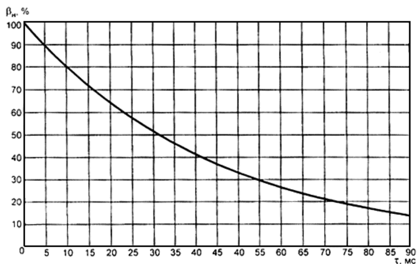
Рисунок 3 - Содержание аperiodической составляющей в процентах
