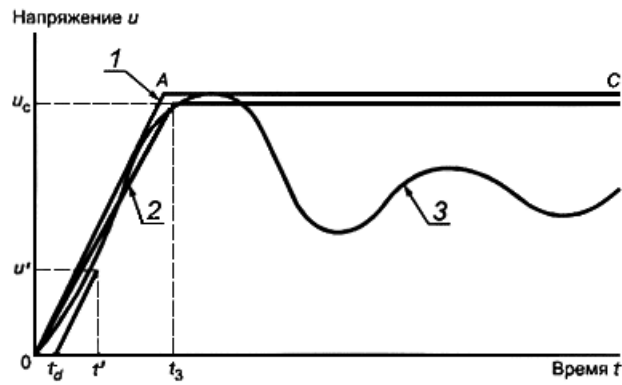
Рисунок 7 - Построение огибающей ПВН, определяемого двумя параметрами
