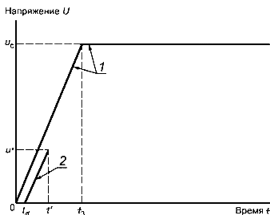
Рисунок 4 - Нормированные характеристики ПВН, определяемого двумя параметрами
