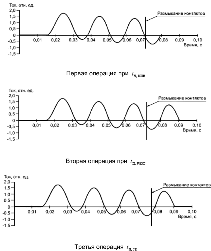
Рисунок 14 - Регулирование моментов инициирования тока и размыкания контактов при однополюсном отключении тока в режиме Т100а выключателями с U_{\text{ном}} \geq 110 кВ
