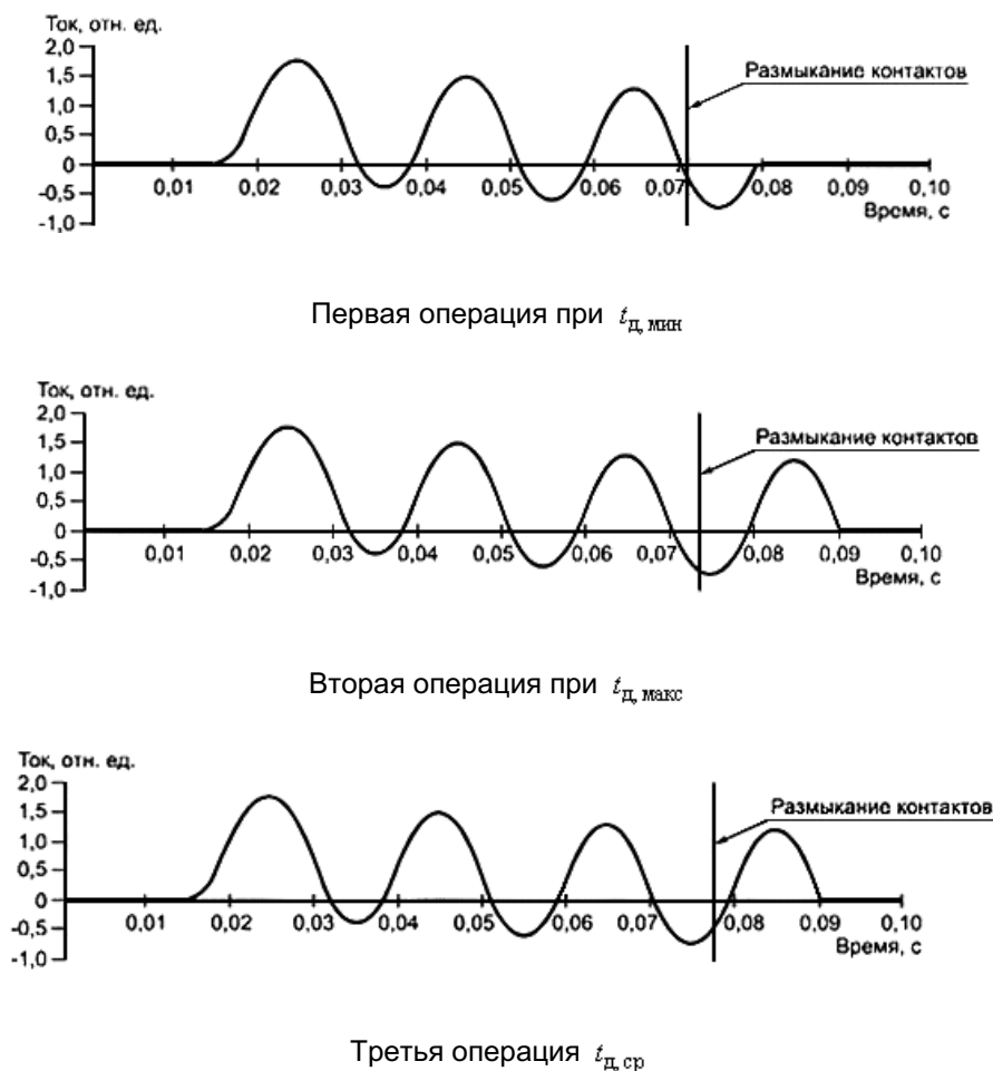
Рисунок 12 - Регулирование моментов инициирования тока и размыкания контактов при однополюсном отключении тока в режиме Т100а выключателями с U_{\text{ном}} \leq 35 кВ
