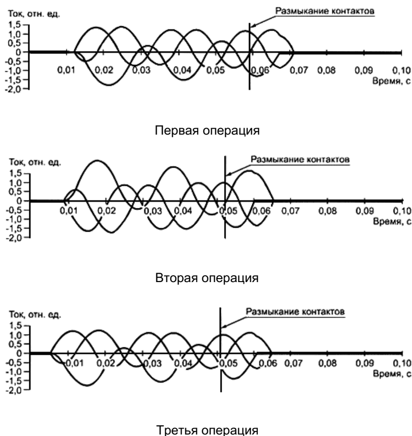
Рисунок 10 - Регулирование моментов инициирования тока и размыкания контактов относительно фазы тока при трехполюсном отключении тока в режиме Т100а
