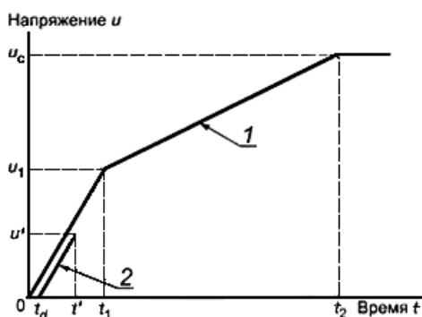
Рисунок 5 - Нормированные характеристики ПВН, определяемого четырьмя параметрами
