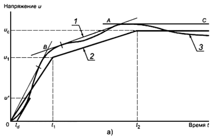
Рисунок 7 - Построение огибающей ПВН, определяемого двумя параметрами
